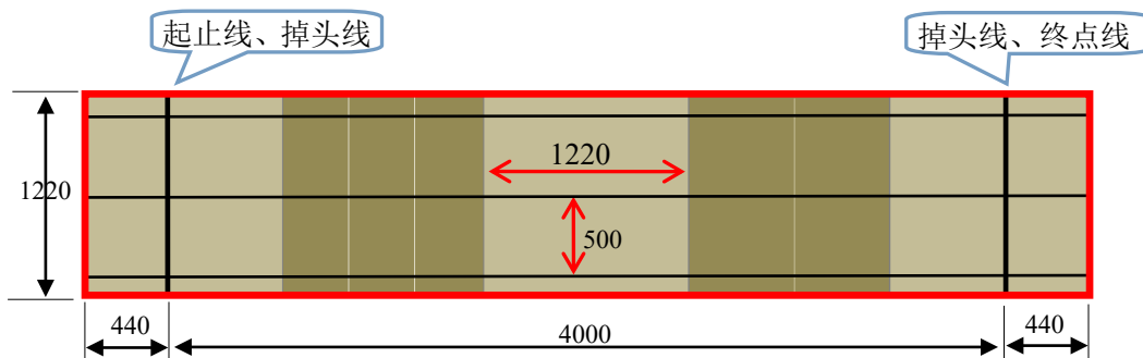
图 1. 双足机器人长短跑障碍跑场地
