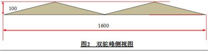
双驼峰侧视图如图 2：长 1600mm，高 100mm，宽 1 米，截面为两个等腰三角形。
